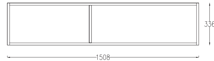
WALL SUSPENDED MODULE WITH DOOR HÄNGENDE TÜRMODULE DEPTH / TIEFE = 350 MM
