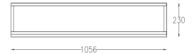
BASE CABINETS GRUNDKOMMODEN DEPTH / TIEFE = 450 MM
