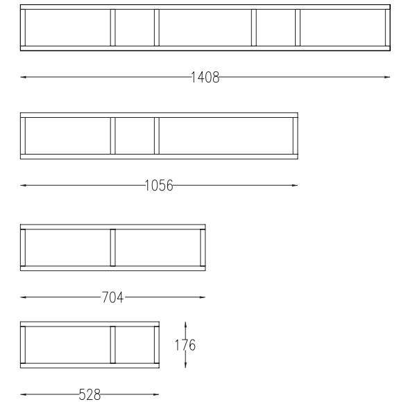
WALL SUSPENDED MODULE WITHOUT DOOR HÄNGEMODULE OHNE TÜR DEPTH / TIEFE = 332 MM
